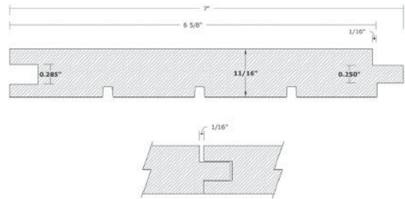
A&BTR CVG Cedar 1X8 T&G 1/16" Fineline
