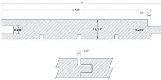
A&BTR CVG Cedar 1X8 T&G 1/8" Fineline
