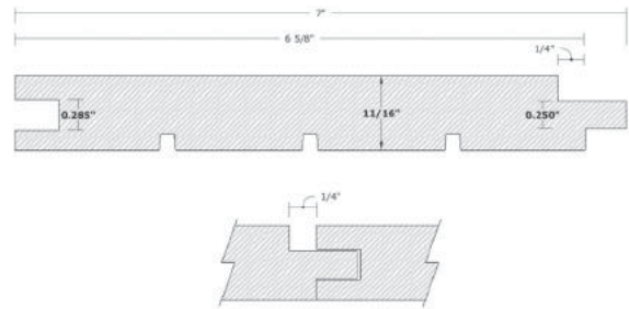
A&BTR CVG Cedar 1X8 T&G 1/4" Fineline
