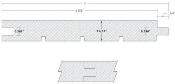
A&BTR CVG Cedar 1X8 T&G Tight
