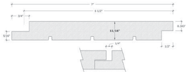
A&BTR CVG Cedar 1X8 Shiplap 1/4" Gap
