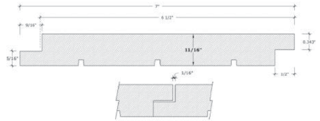
A&BTR CVG Cedar 1X8 Shiplap 1/16" Gap
